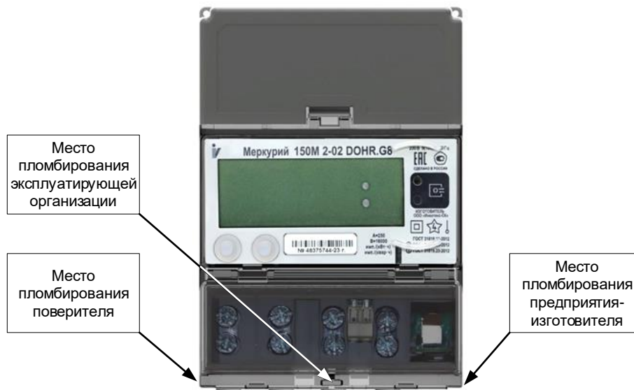
Рисунок 4.1 – Вид счетчиков Меркурий 150М, Меркурий 150, Меркурий 150Х с указанием мест пломбирования
